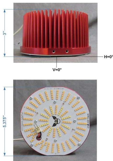
FIG. 1 LUMINAIRE
